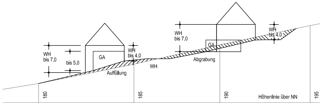
GELÄNDESCHNITT M 1 : 500
